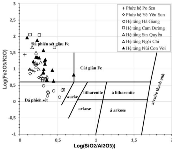
Hình 3. Biểu đồ tỷ lệ \text{SiO}_2/\text{Al}_2\text{O}_3 với \text{Fe}_2\text{O}_3/\text{K}_2\text{O} (Herron, 1988).
