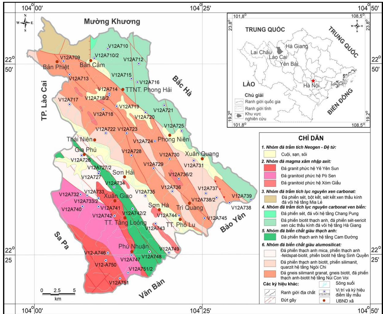
Hình 1. Sơ đồ địa chất thạch học và vị trí lấy mẫu đất tầng mặt khu vực huyện Bảo Thắng, tỉnh Lào Cai (thành lập từ bản đồ địa chất tỷ lệ 1:200.000 tờ Bắc Quang do Trần (chủ biên), 1988; Đình và Phạm (hiệu đính), 1994).
