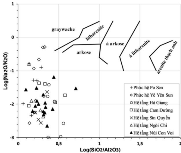
Hình 2. Biểu đồ tỷ lệ \text{SiO}_2/\text{Al}_2\text{O}_3 với \text{Na}_2\text{O}/\text{K}_2\text{O} (Pettjohn và nnk., 1972).
